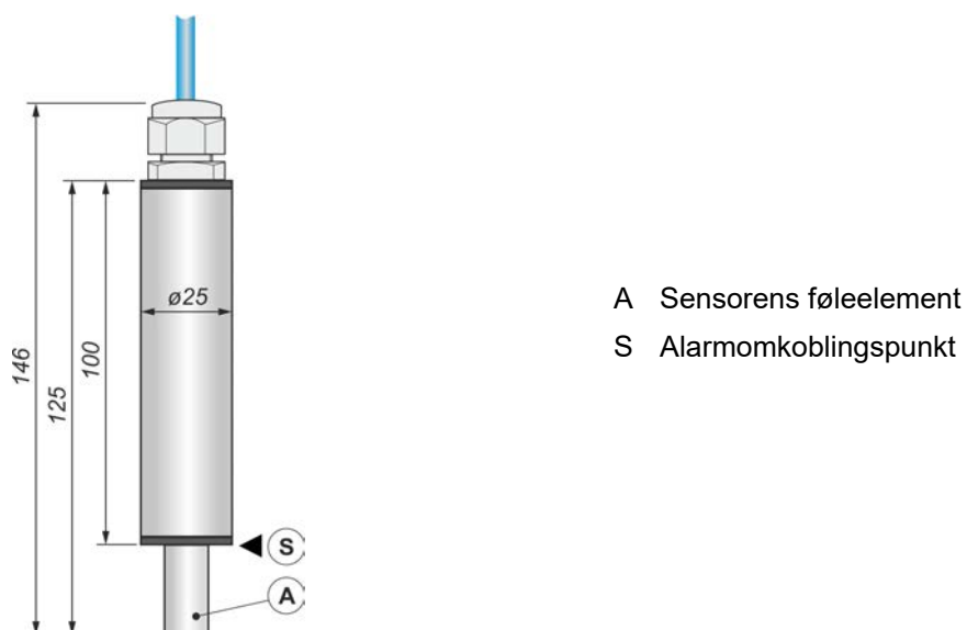
Figur 3. idOil-LIQ-sensor til højt væskenniveau – struktur og mål (mm)
