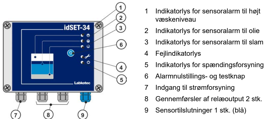
Figur 17. idSET-34-kontrolenhedens funktioner
