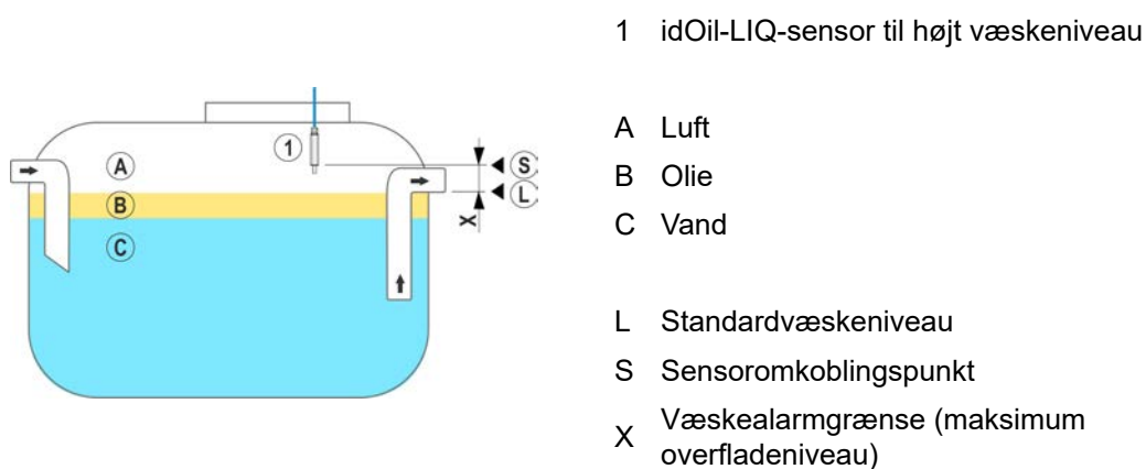
Figur 10. Installation af idOil-LIQ-sensor til høj væskegrænse
