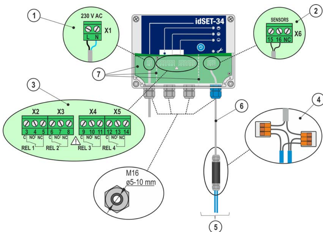
Figur 14. Tilslutning med en to-sensorkabelkonnektor LCJ1-2
