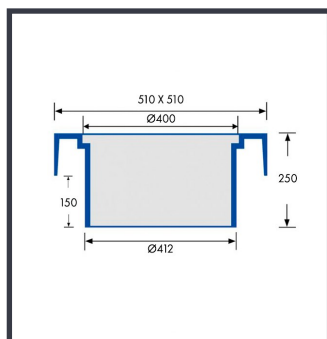
ECO-425-CS D400 Firkantet karm & dæksel VVS nr.: 22.1119.242
