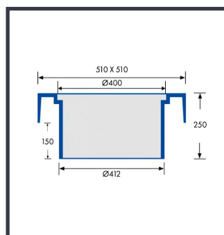
ECO-425-GS D400 Firkantet karm & rist VVS nr.: 22.1119.742
