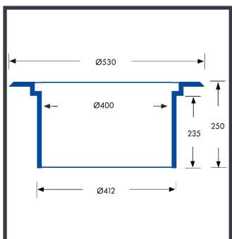
ECO-425-CR D400 Rund karm & dæksel VVS nr.: 22.1117.142
