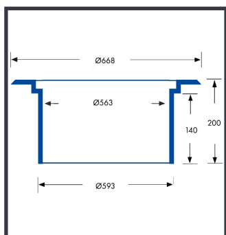
ECO-600-CR D400 Rund karm & dæksel VVS nr.: 22.1117.160
