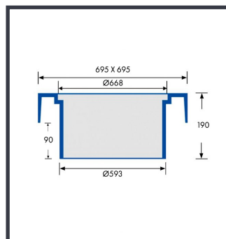
ECO-600-GS D400 Firkantet karm & rist VVS nr.: 22.1119.760
