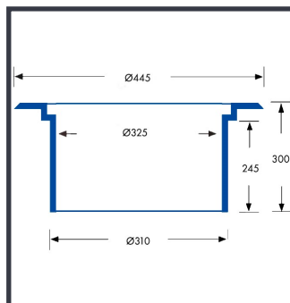
ECO-315-CR D400 Rund karm & dæksel VVS nr.: 22.1117.131
