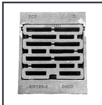
ECO315-RTL5 Rendestensrist VVS nr.: 22.1129.831
