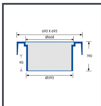
ECO-600-CS D400 Firkantet karm & dæksel VVS nr.: 22.1119.260
