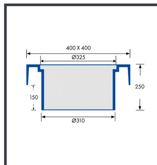
ECO-315-CS D400 Firkantet karm & dæksel VVS nr.: 22.1119.231
