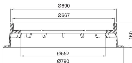
Ø600 Fast karm 16 cm
