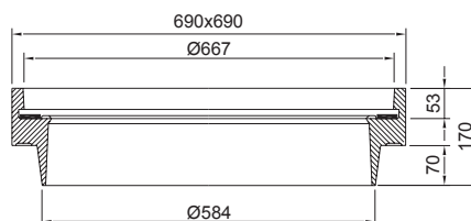
Ø600 Firkantkarm
