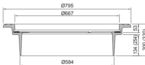
Ø600 Flydekarm Med inspektionsslider 320 mm. ved langt skørt
