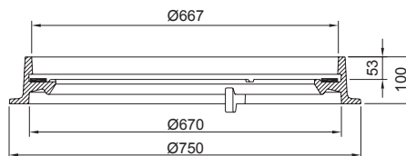
Ø600 Fast karm 10 cm
